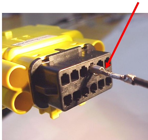
180° Mis-orientation
