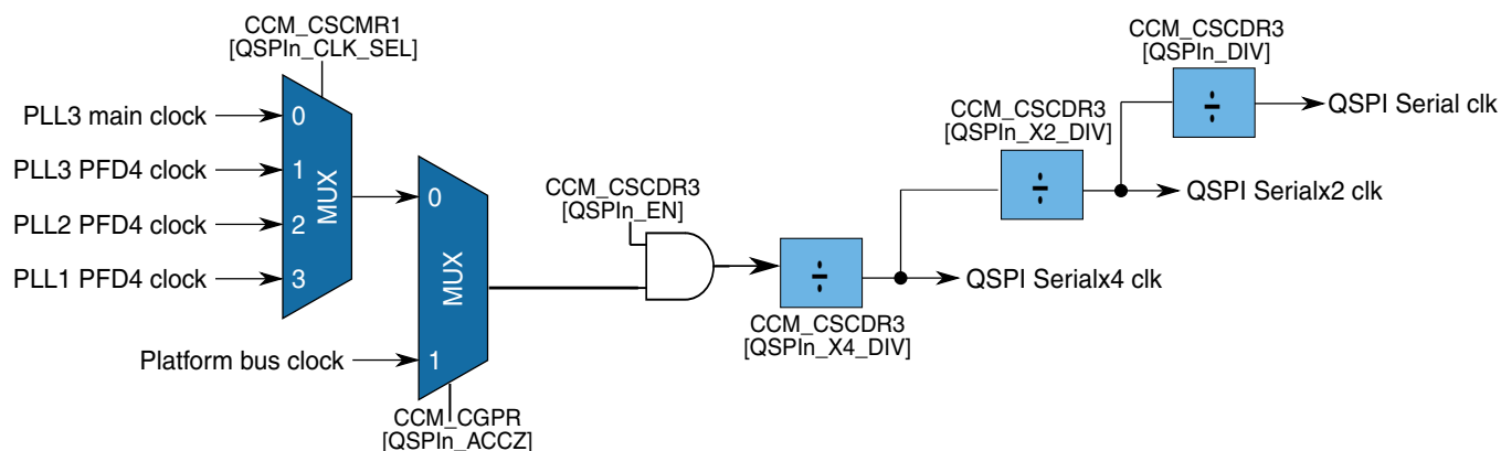
Figure 9-4. QuadSPI Clocking
