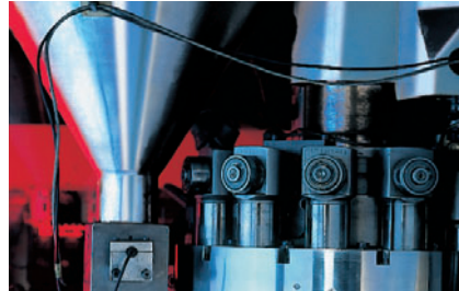
Vollautomatische Rundläuferpresse
